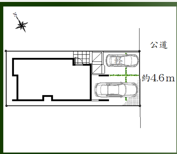
配置図
