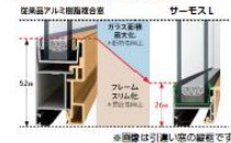
※図例は引違い窓の縦断です。
