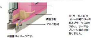
※1サモスL-H（レール固定バー枠）およびサモスLの下部は、サマルブレイク構造ではありません。
